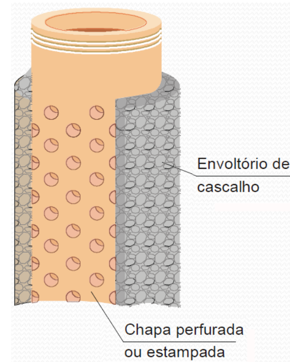
Filtros com envoltório de cascalho
